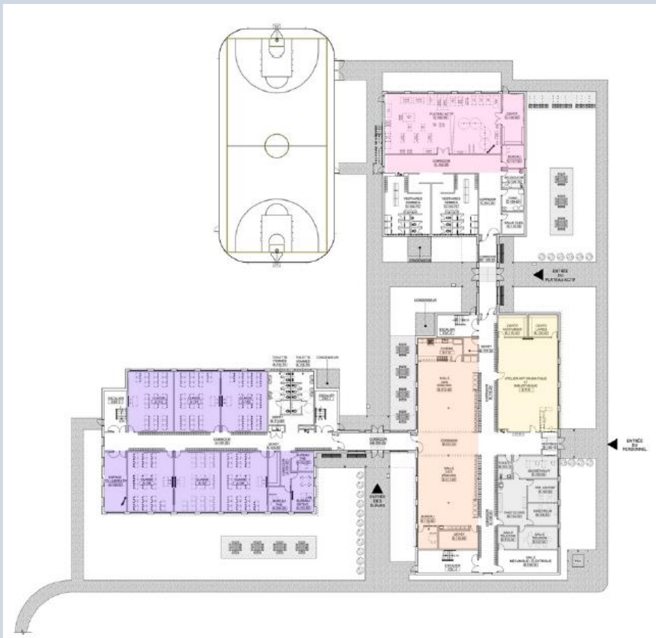
Rez-de-chaussée
